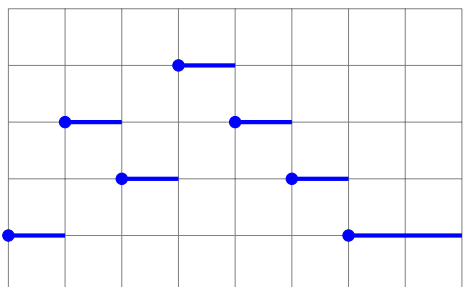
Hill: (C,1) / (E,1) \setminus (D,1) / (F,1) \setminus (E,1) \setminus (D,1) \setminus (C,2)
