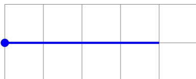
mms1: (C,4)
